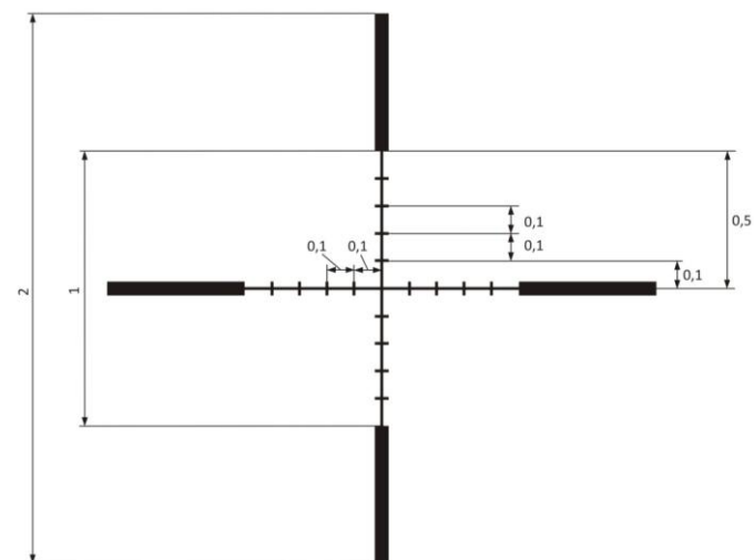
Рисунок 33 – Прицельная сетка (размер в м/100м дистанции)
